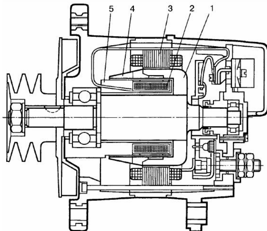
Рис. 1.12. Бесконтактный генератор:
