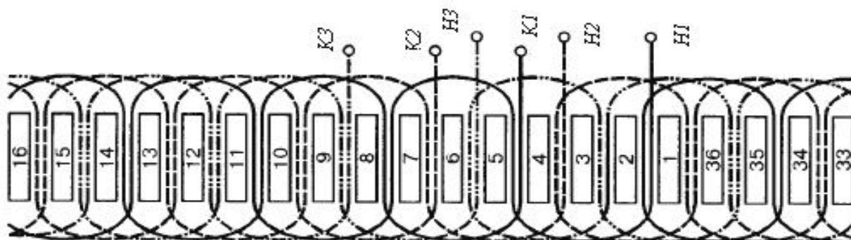
Рис. 1.8. Волновая обмотка якоря при соединении фаз в звезду, Z = 36 :
