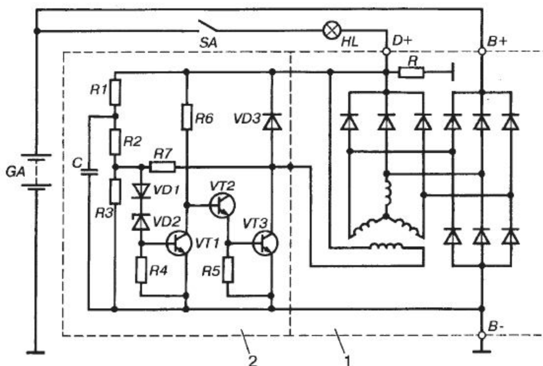
Рис. 1.21. Схема регулятора напряжения EE 14V3 фирмы Bosch : 1 – генератор, 2 – регулятор напряжения, SA – выключатель зажигания, HL – лампа контроля работоспособного состояния генераторной установки
