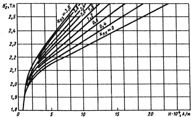
Рис. III. Кривые намагничивания стали марки 2013
