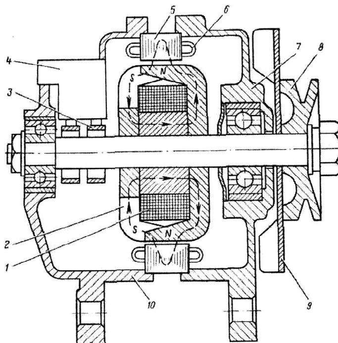
Рис. 1.1. Конструкция автомобильного генератора переменного тока:
