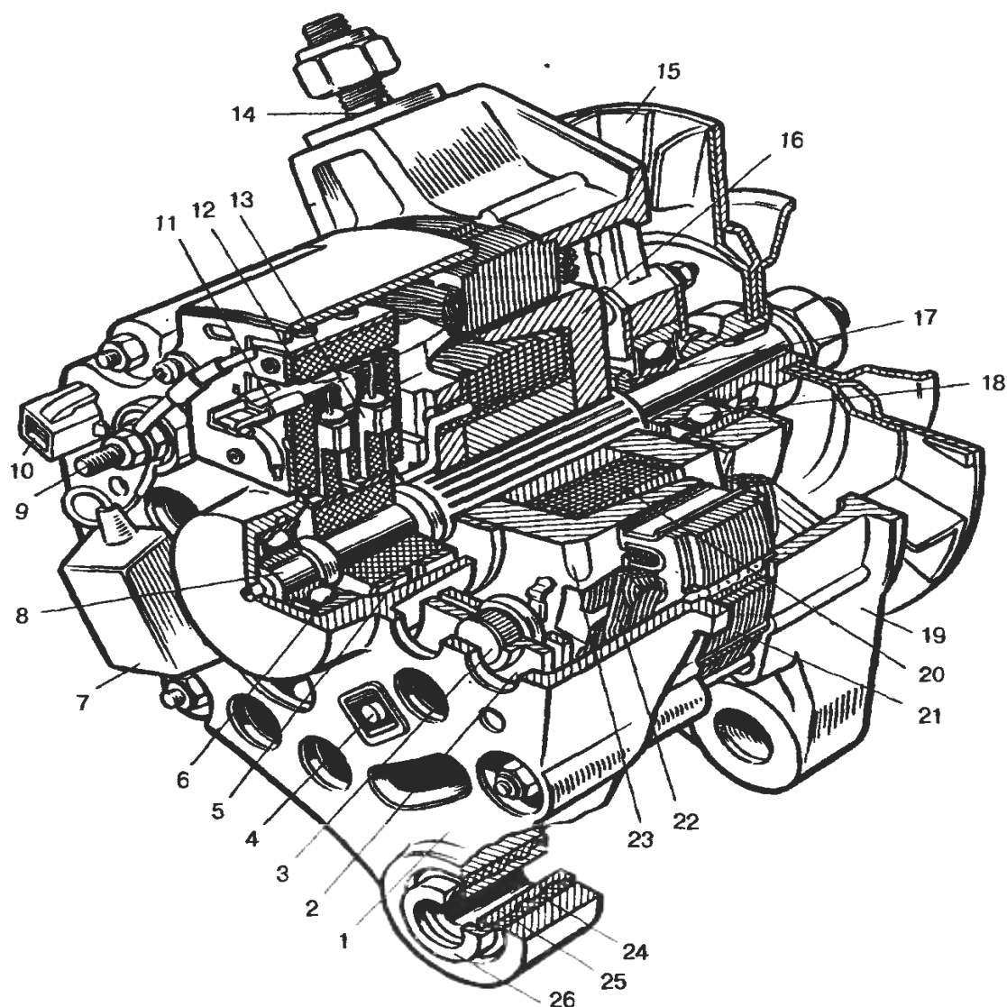
Рис. 1.3. Генератор традиционной конструкции:
