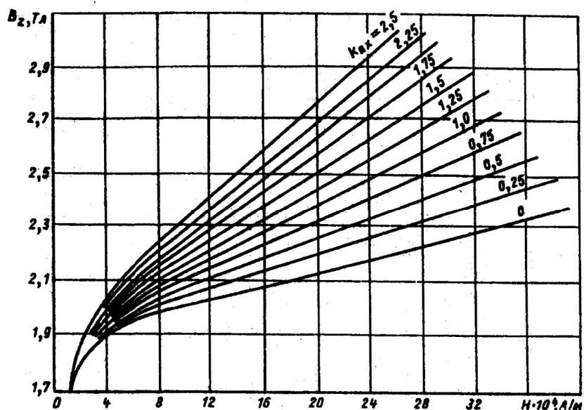
Рис. П4. Кривые намагничивания стали марки 1411
