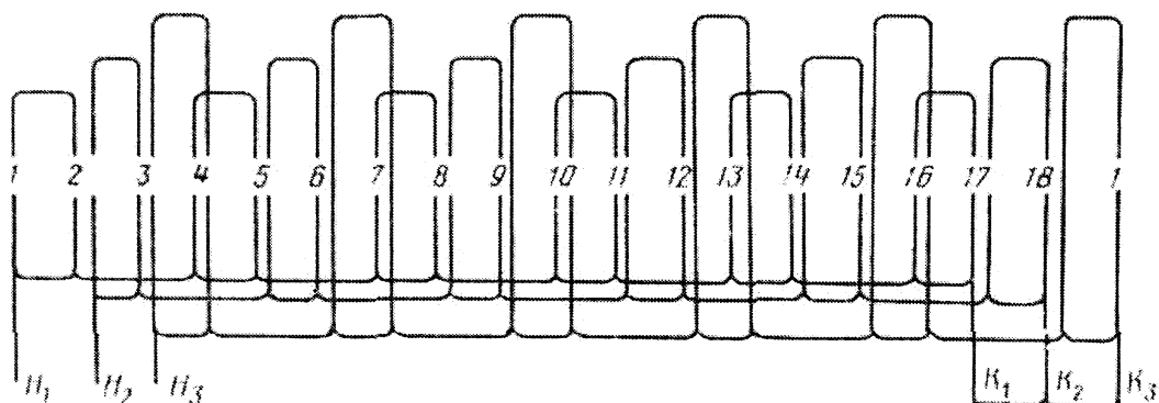
Рис. 1.7. Обмотка якоря при соединении фаз в звезду, Z = 18 :
