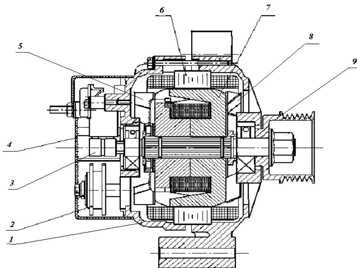
Рис. 1.4. Генератор компактной конструкции 94.3701: 1 – задняя крышка; 2 – блок выпрямителей; 3 – контактные кольца; 4 – пластмассовый кожух; 5, 8 – вентиляторы; 6 – статор; 7 – ротор; 9 – шкив
