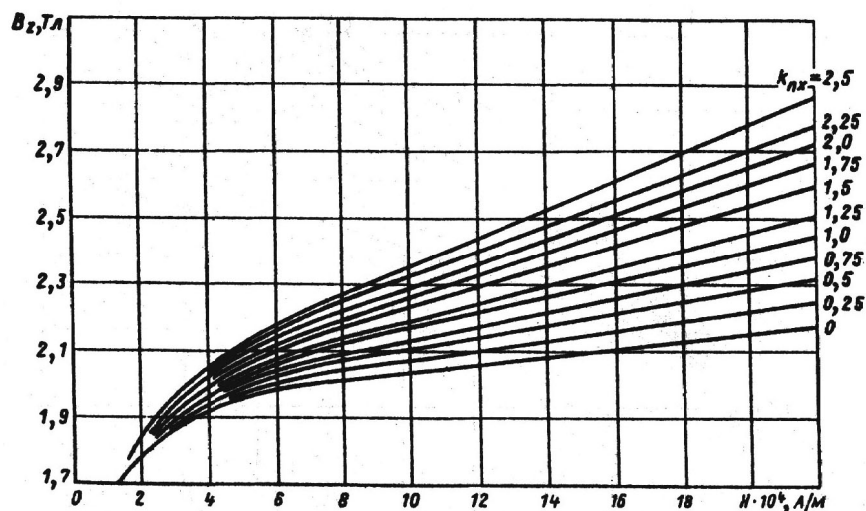
Рис. П5. Кривые намагничивания стали марок 1511, 1512, 1513 (к определению магнитного напряжения зубцовых зон машин постоянного тока и синхронных)
