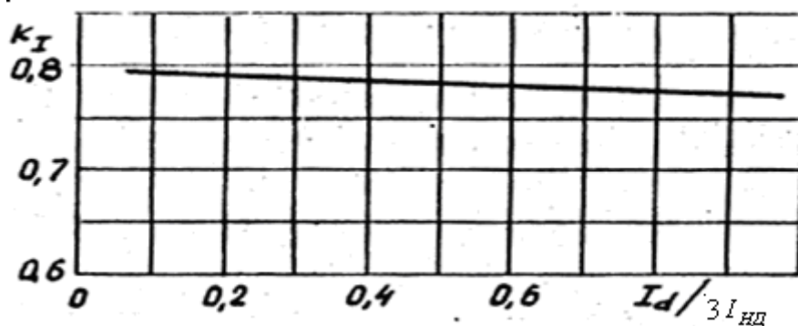
Рис. 2.4. Зависимость K_I = f\left(\frac{I_d}{3I_{нд}}\right) .
